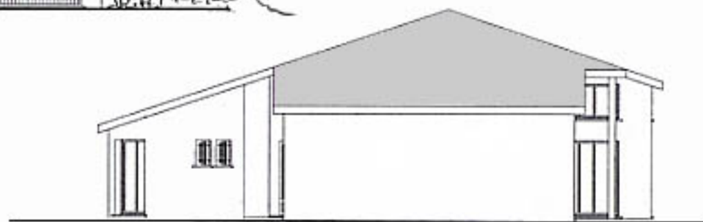
FAÇADE NORD
