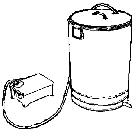
Figure 24 : Extracteur de la cire à la vapeur
