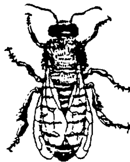
Figure 25 : Abeille ouvrière
