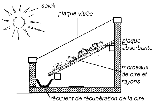
Figure 22 : Cérificateur solaire
