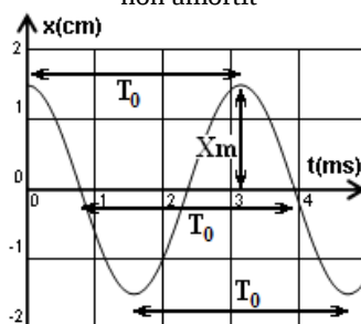
Oscillateur libre et harmonique
