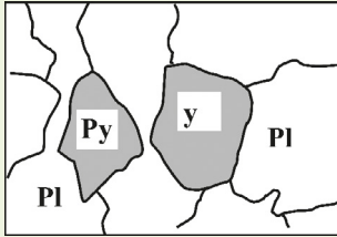
Gabbro : origine des métagabbros
