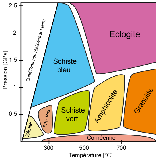
Diagramme P - T des faciès métamorphiques et leurs domaines de stabilité
