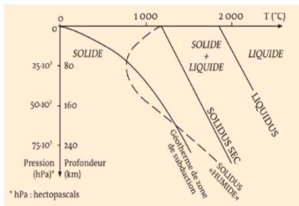
Diagramme pression/ température
