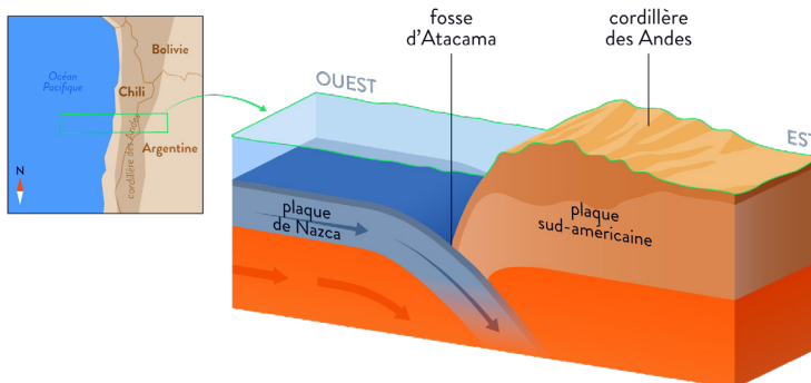
Coupe topologique réalisée dans la zone de subduction
